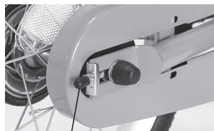
チェーン引きのボルト(黒いカバー付) ※黒いカバーがついていないインチもあります。
