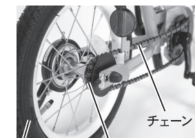
後輪 フリーギア チェーン
