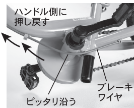
上から見た図 ブレーキワイヤの位置に注意
